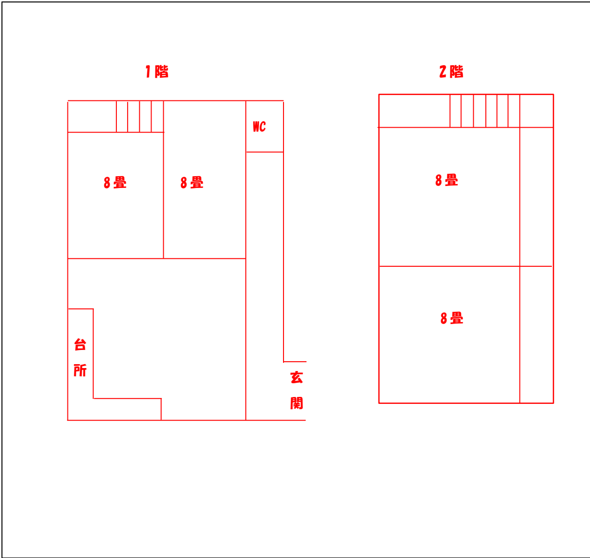
間取り略図
